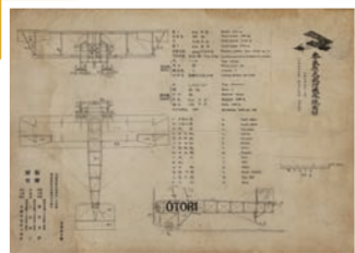
明治四十五年四月川崎馬見場にて飛行セシ奈良原式 最初ノ飛行機ノ図解
